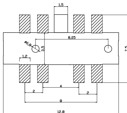
P.C.B端子位置
